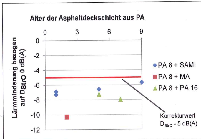
Abbildung 5: Lärm mildernde Wirkung verschiedener Asphaltdeckschichten aus Offenporigem Asphalt auf der A 2 in Abhängigkeit des Alters (Ergebnisse aus SPB Einzelmessungen)
