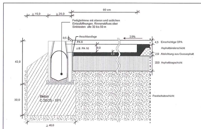
Abbildung 2: Beispiel für einen seitlichen Abfluss mit einer Kastenrinne aus Polymerbeton, Maße in cm
