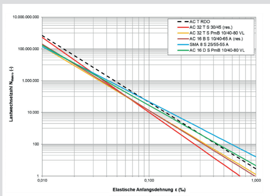
Bild 4: Ermüdungsfunktionen der Asphalte, die für die rechnerischen Dimensionierungen in den folgenden Abschnitten genutzt wurden
