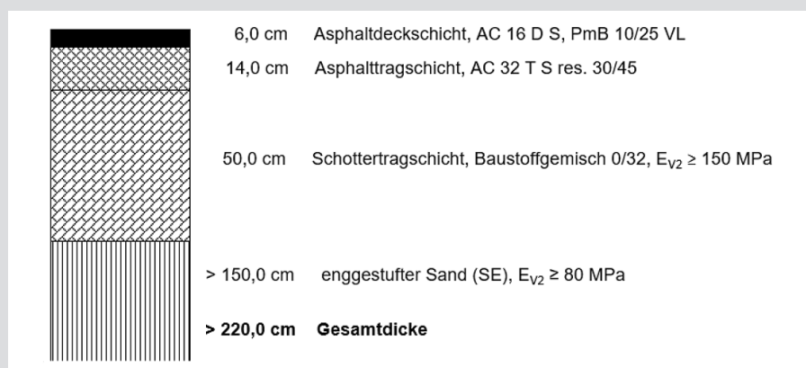
Bild 10: Aufbau der Verkehrsflächenbefestigung für die Deichquerung
