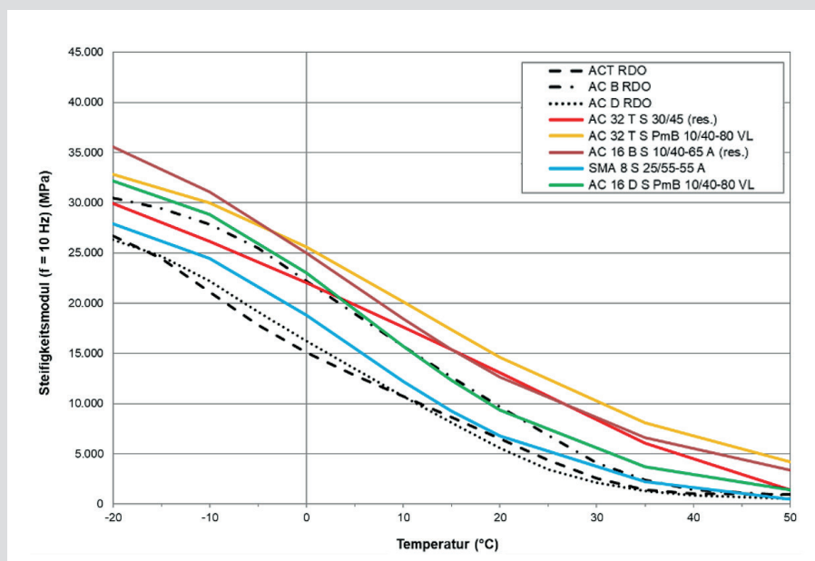
Bild 3: Steifigkeits-Temperaturfunktionen der Asphalte, die für die rechnerischen Dimensionierungen in den folgenden Abschnitten genutzt wurden
