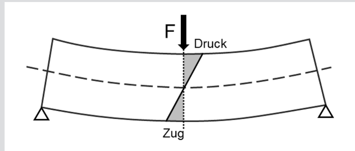
Bild 2: Spannungsverlauf eines Biegebalkens bei vollem Verbund der Schichten
