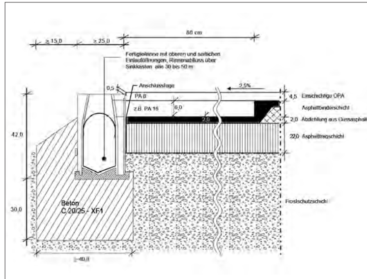
Bild 8: Beispiel für einen seitlichen Abfluss mit einer Kastennrinne aus Polymerbeton, Maße in cm [1]
